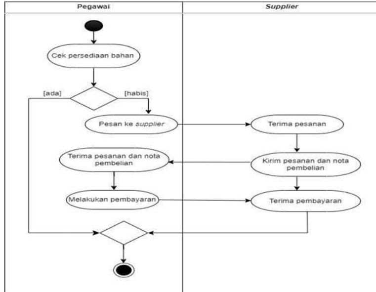
Gambar 2. Activity Diagram Pembelian pada Ade Laundry
